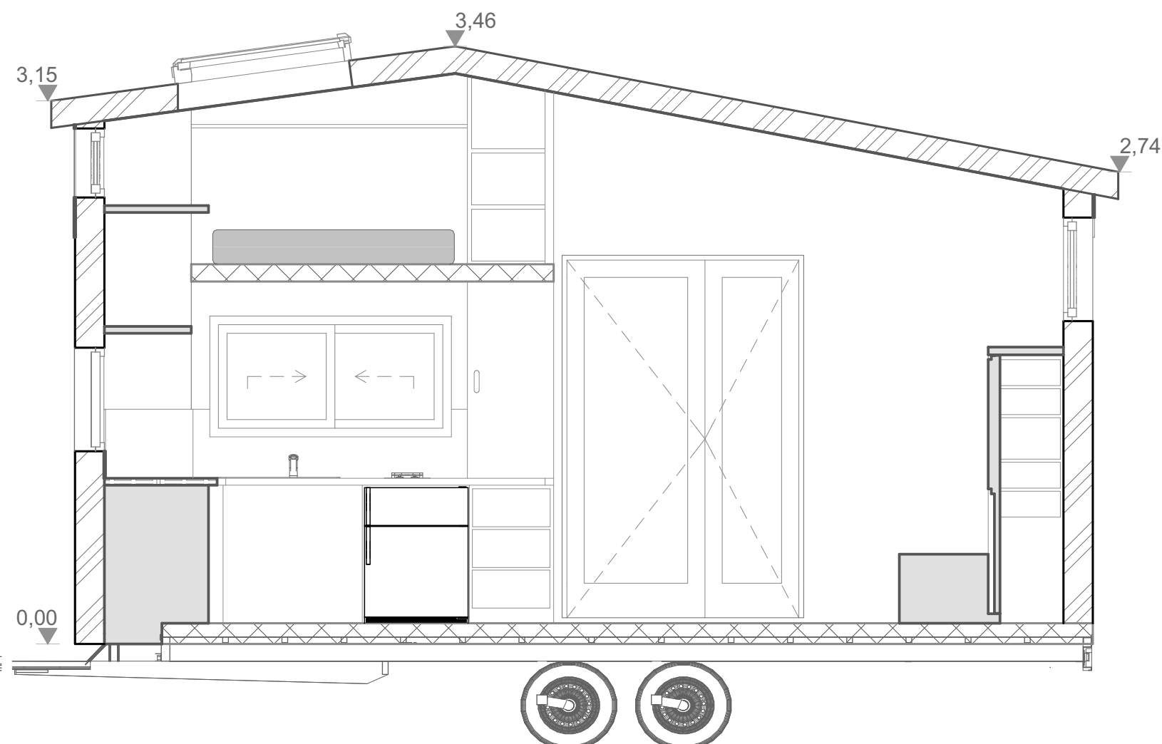
Coupe BB
