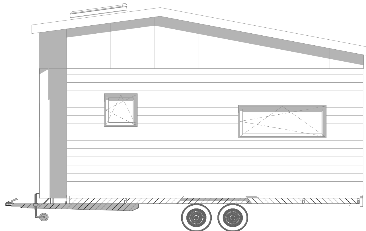
Façade Nord
