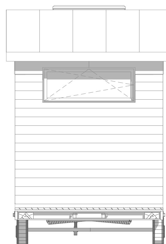
Façade Ouest
