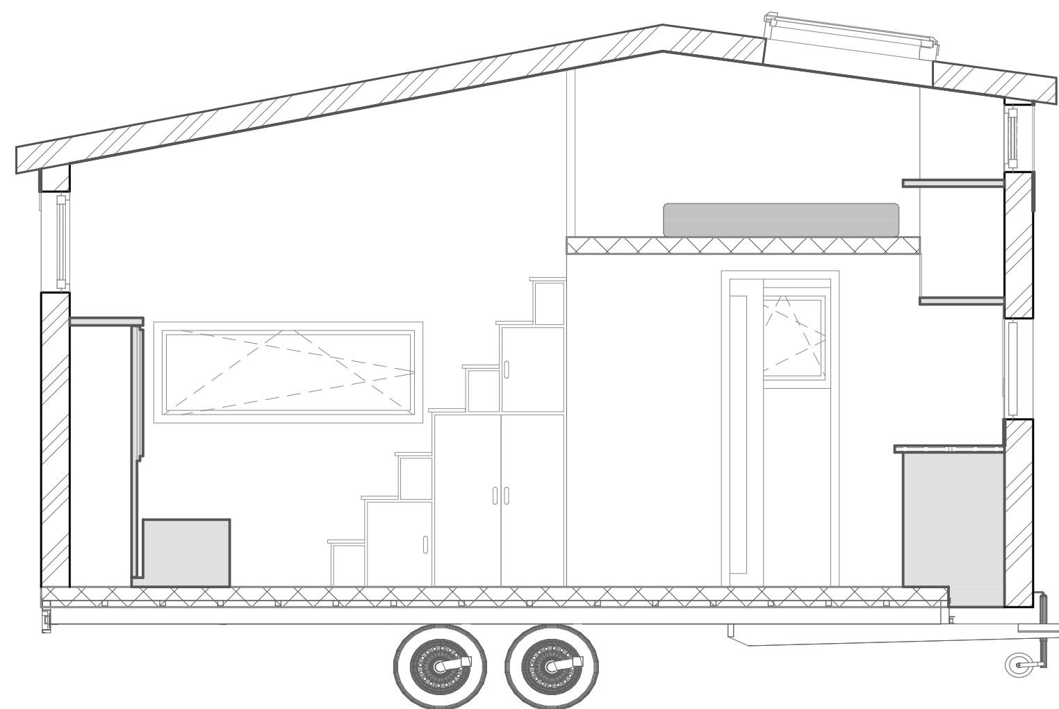
Coupe AA
