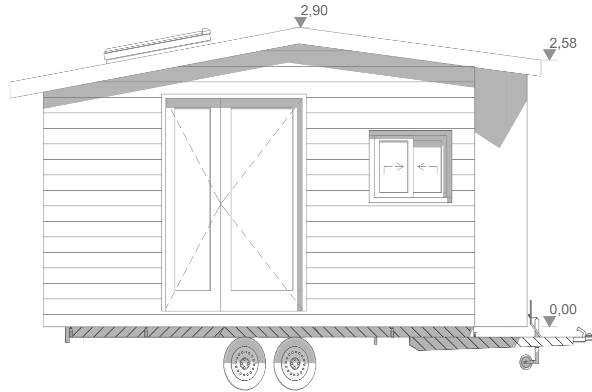
Façade Est
