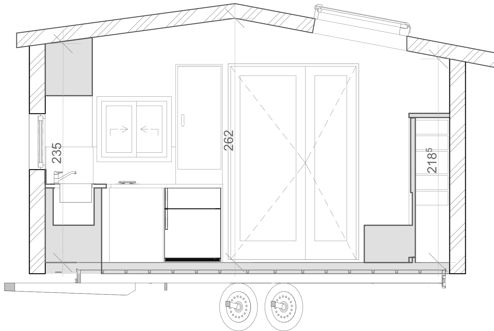
Coupe AA
