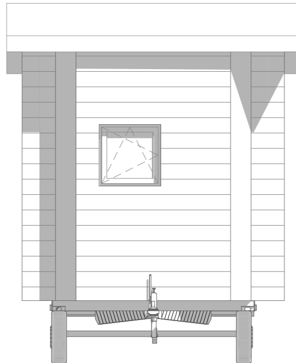
Façade Est
