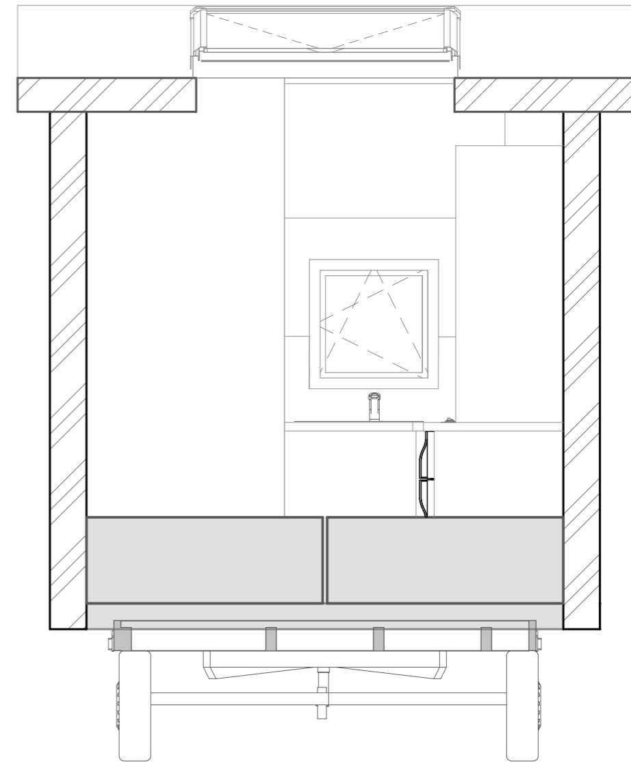
Coupe BB
